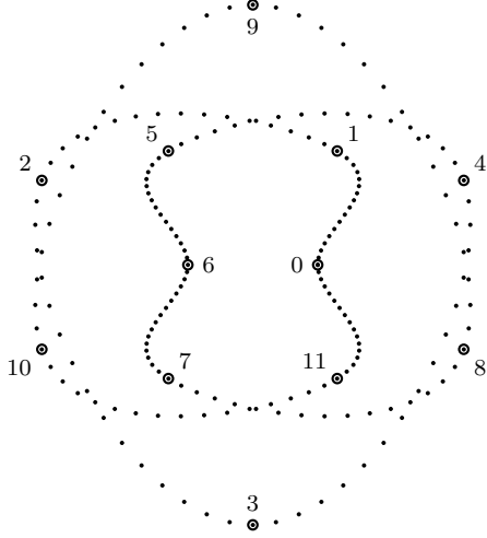
Рис. 1. Точки интерполяции и значения сплайна
