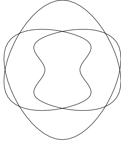
Рис. 2. Замкнутая ломаная
